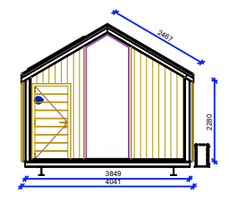
ACHTERZIJDE
