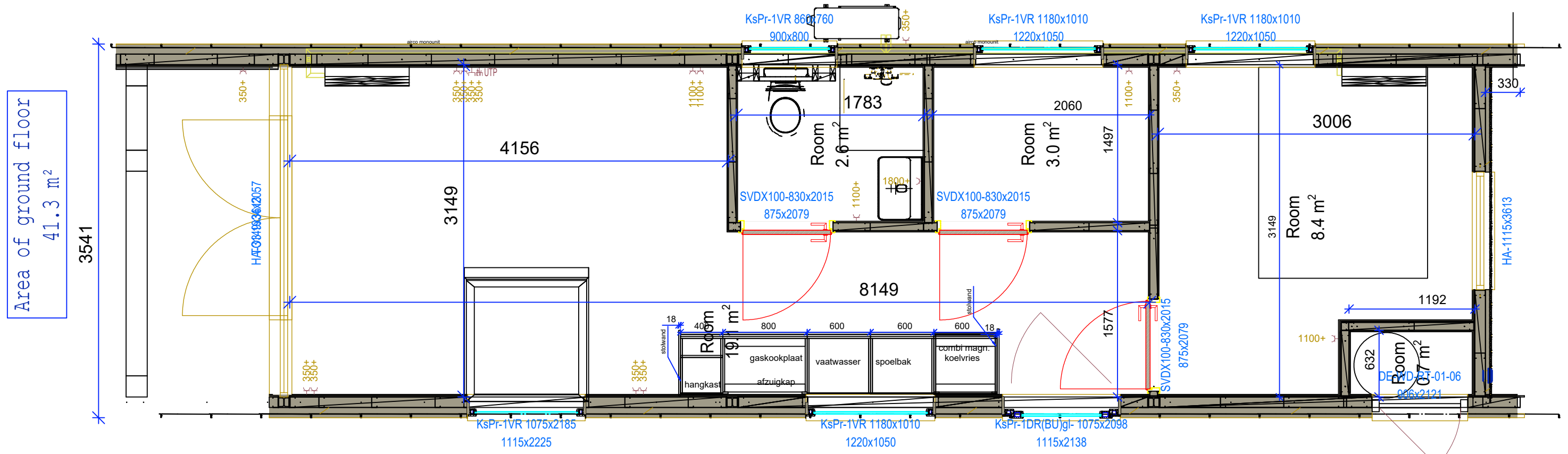
PLATTEGROND
